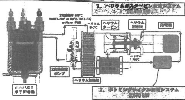
図2 二次系ループ及び発電システムの概要
