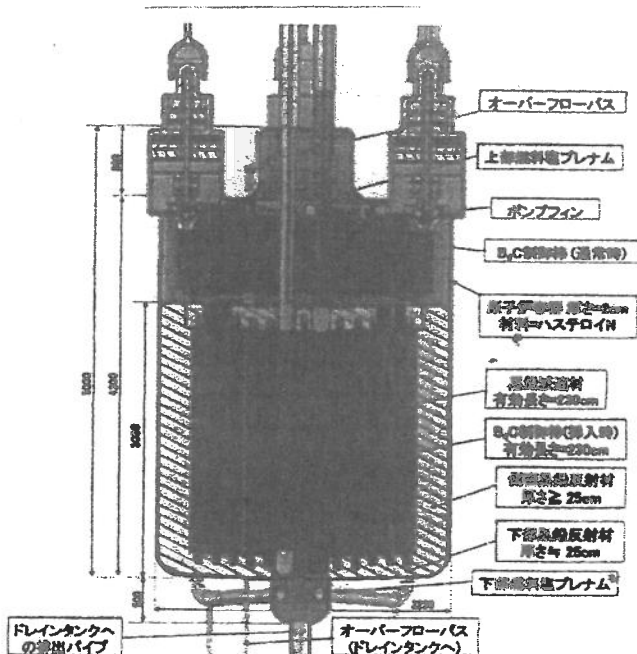
図5 超小型熔融塩炉 miniFUJI II の断面図
